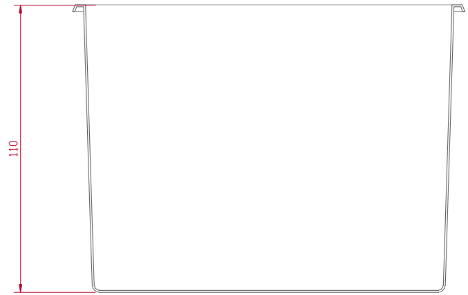
SECCIÓN A-A'
