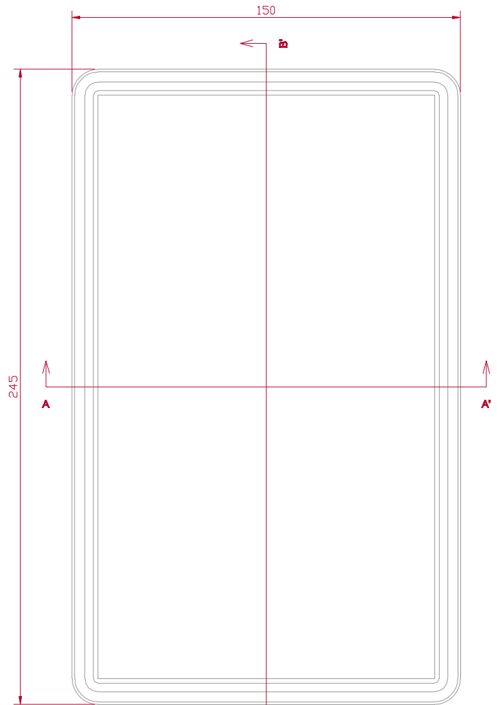
PLANTA
