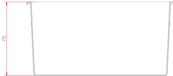
SECCIÓN A-A'
