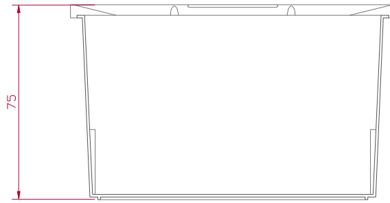
SECCIÓN A-A'
