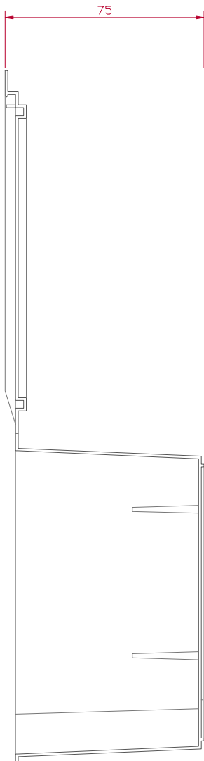
SECCIÓN B-B'
