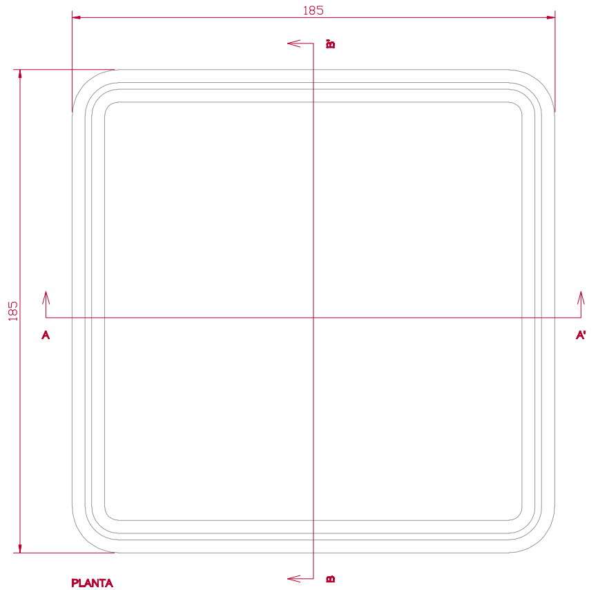
PLANTA
