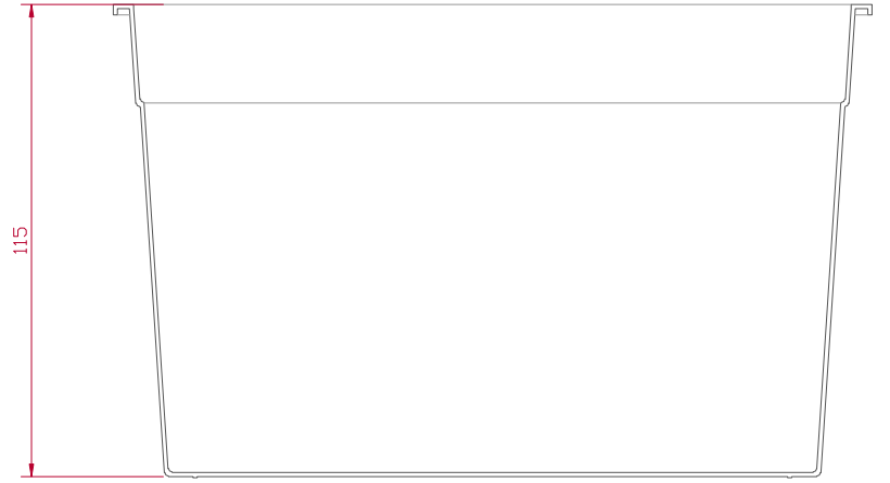
SECCIÓN A-A'
