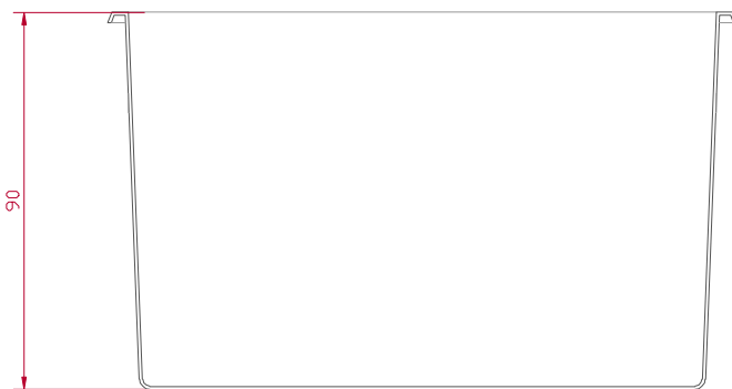
SECCIÓN A-A'
