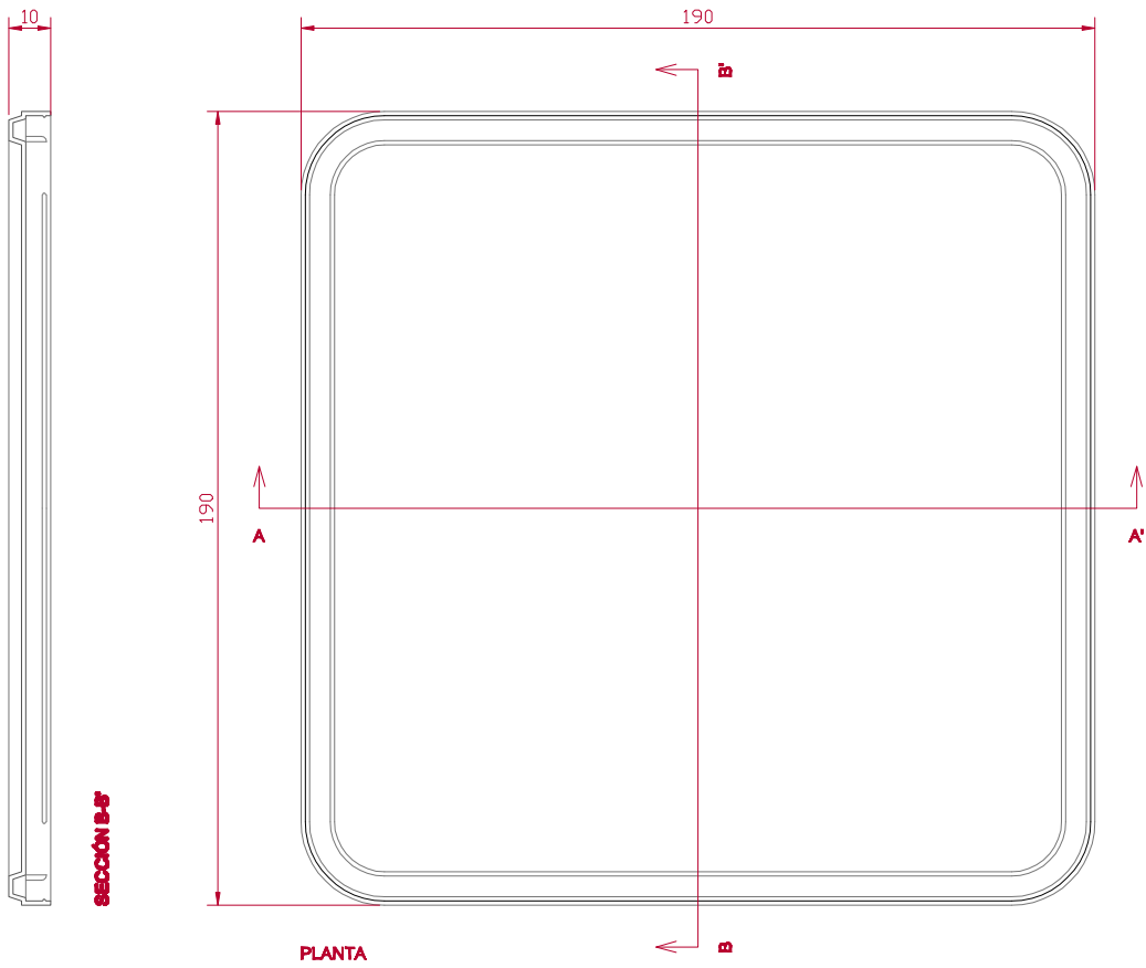
TAPA TARRO CUADRADO ESCALA 1:2
