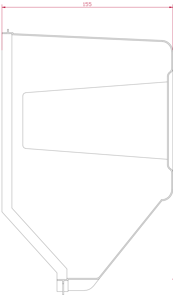
SECCIÓN B-B'
