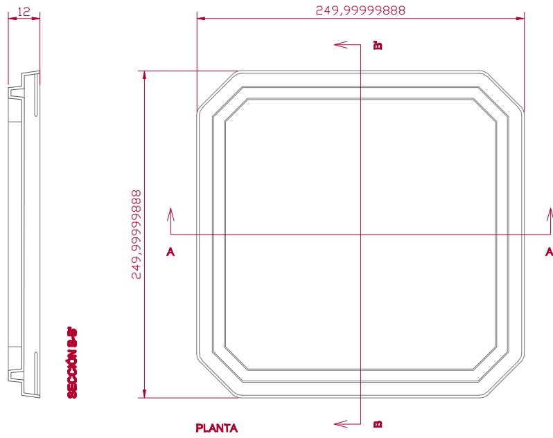
TAPA CAJA CON CHAFLÁN ESCALA 1:2
